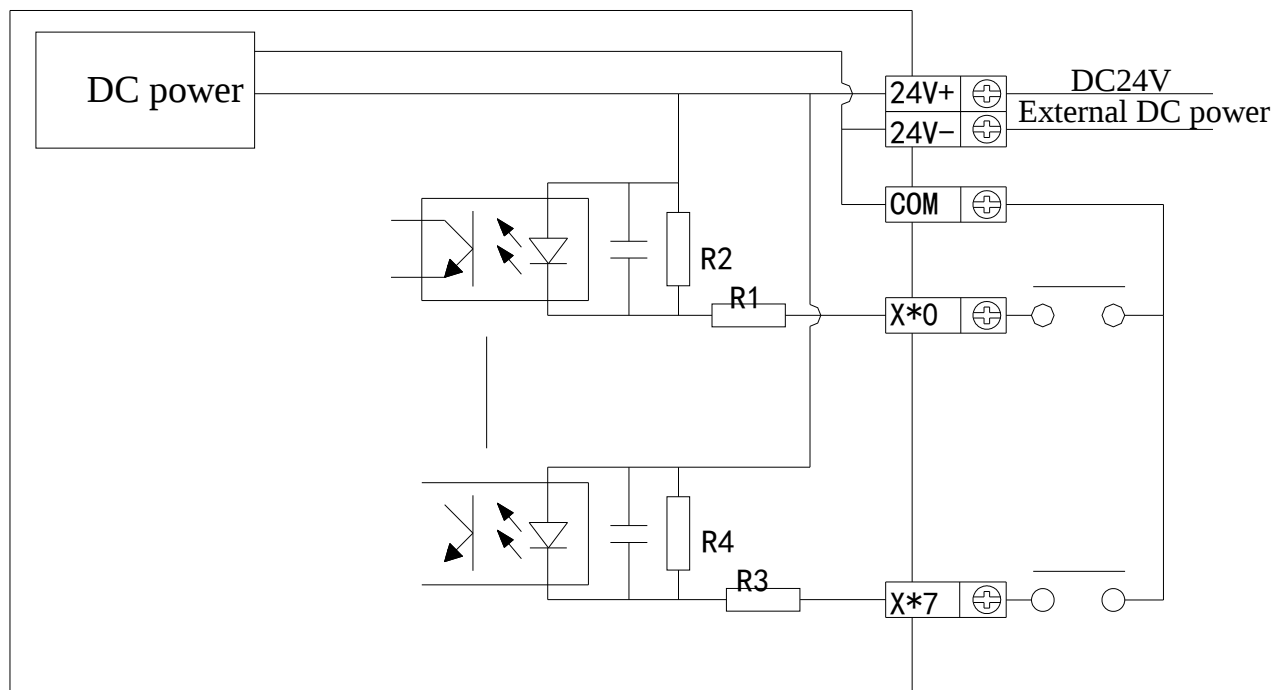
NPN type
