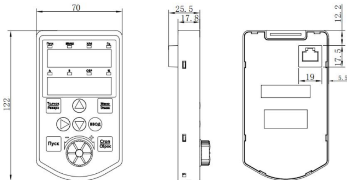
Рисунок 3-6 Габаритные размеры внешней панели управления
