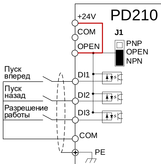
Рисунок 5-7 Типовое подключение и настройки ПЧ Трехпроводный режим 1
