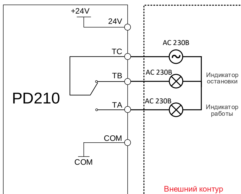
Рисунок 4-17 Схема подключения выходного реле
