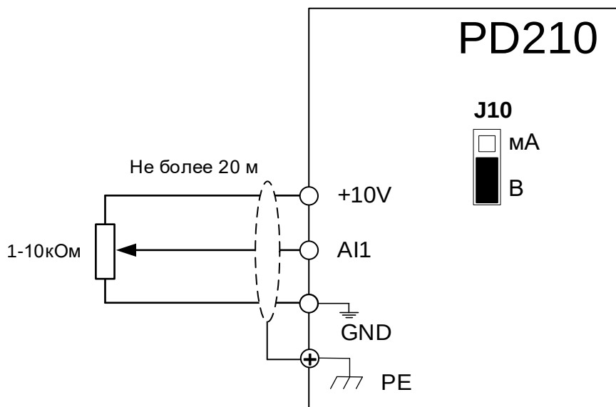
Рисунок 4-14 Схема подключения аналоговых сигналов в режиме напряжения
