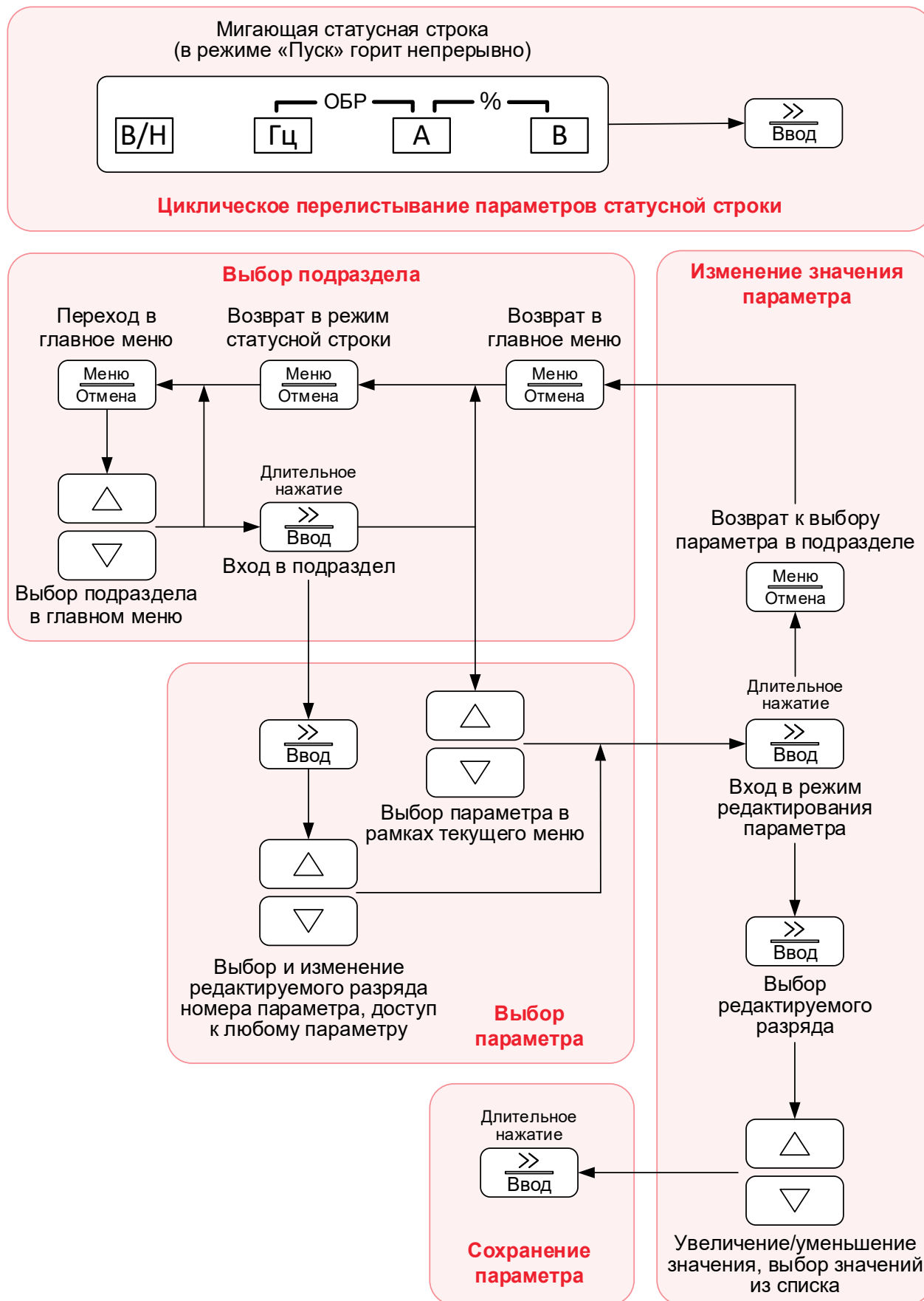
Рисунок 5-2 Навигация и настройка параметров
