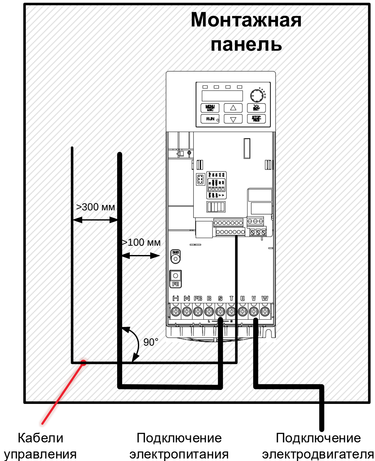
Рисунок 4-3 Схема прокладки силовых и сигнальных кабелей
