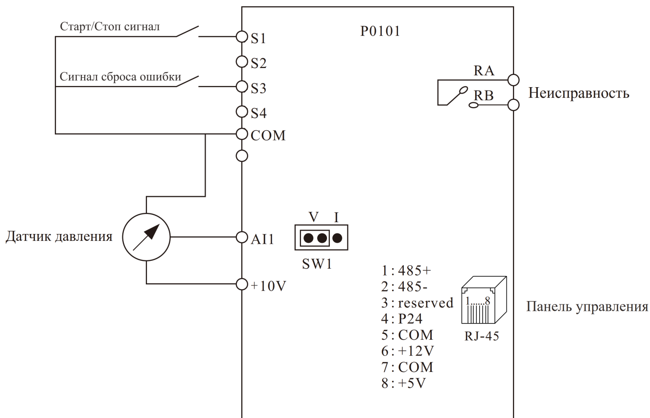
Схема подключения к насосу для настройки управления с поддержанием постоянного давления
