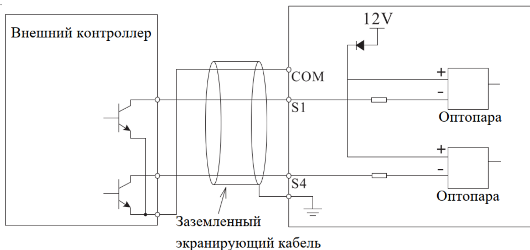
Подключение цифровых входных клемм
