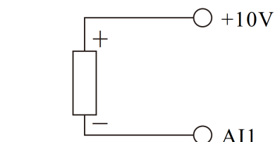
Датчик давления с двухпроводным подключением
