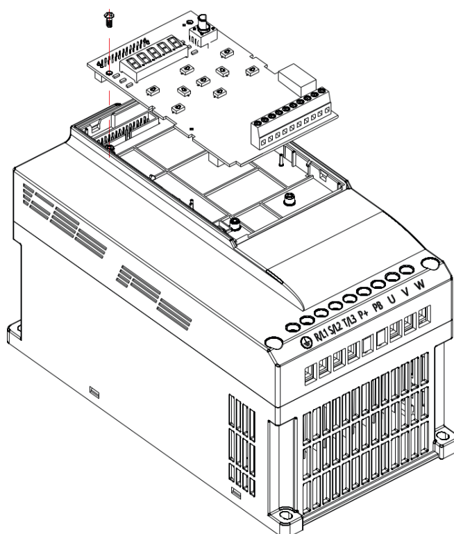
Стандартная плата управления P0100: внешний вид и установка
