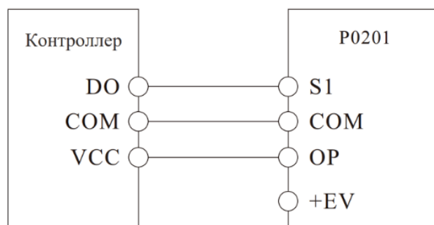
NPN тип (внешнее питание)
