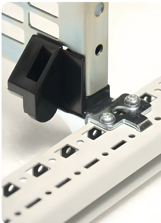
Крепление монтажной панели MPP.xx.xx.LGE на профиль — низ.
