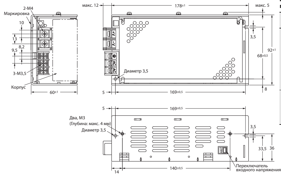
Размеры и диаметры отверстий панельного монтажа
