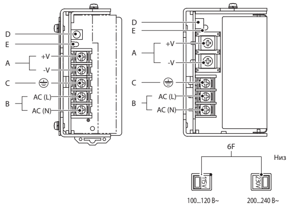
Прим.: Показана модель S8JX-G05024CD
