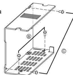
Горизонтальный боковой монтаж
