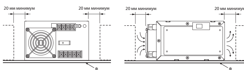
Нижний монтаж
