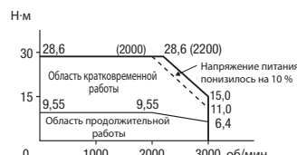
R88M-KH2K020F/C (400 В, 2 кВт)
