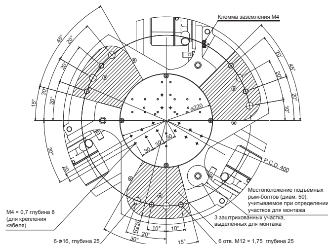
ДЕТАЛИЗАЦИЯ МОНТАЖНОЙ ПОВЕРХНОСТИ
