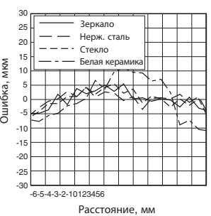
Отражение: стандартное
