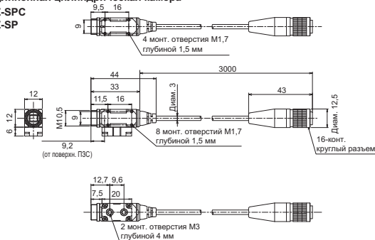
Удлиненная цилиндрическая камера
