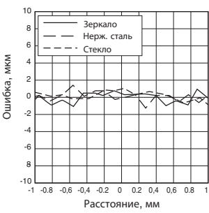
Отражение: зеркальное
