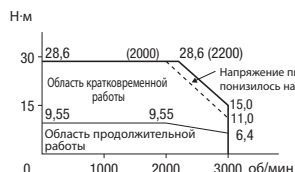
R88M-K2K020F/C (400 В, 2 кВт)
