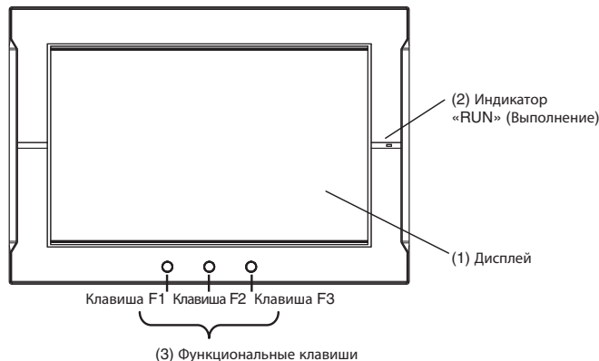
Лицевая панель
