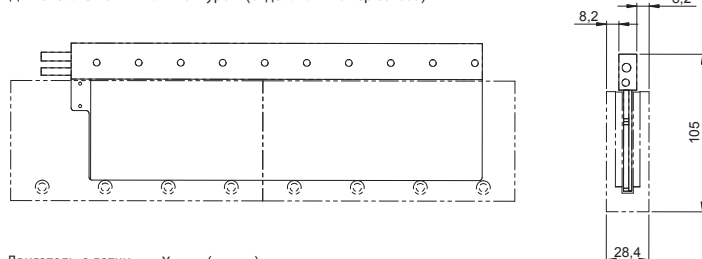
Двигатель с датчиком Холла (опция) L1
