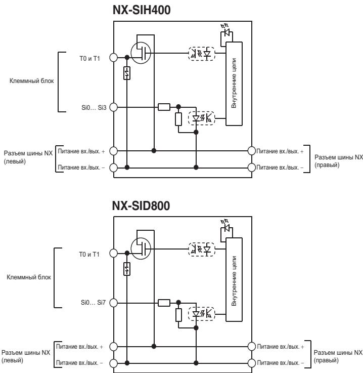
Внутренняя схема
