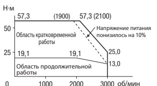
R88M-K4K020F/C (400 В, 4 кВт)
