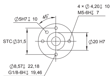
Размеры захватного устройства
