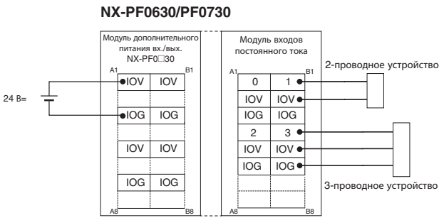
Схема подключения клемм
