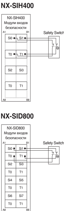
Схема подключения клемм
