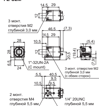
Камера на 2 Мп
