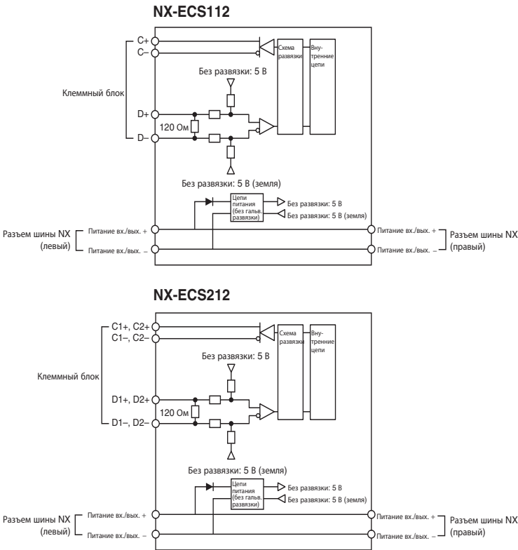
Внутренняя схема
