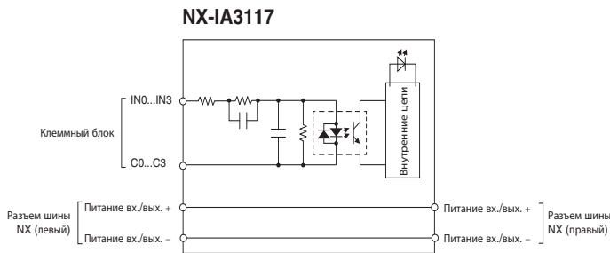
Внутренняя схема
