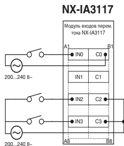
Схема подключения клемм
