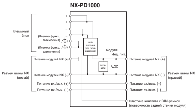
Внутренняя схема
