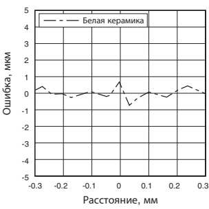
Отражение: диффузное
