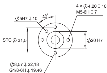
Размеры захватного устройства
