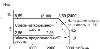
R88M-K60020F/C (400 В, 600 кВт)
