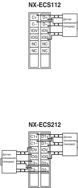
Схема подключения клемм
