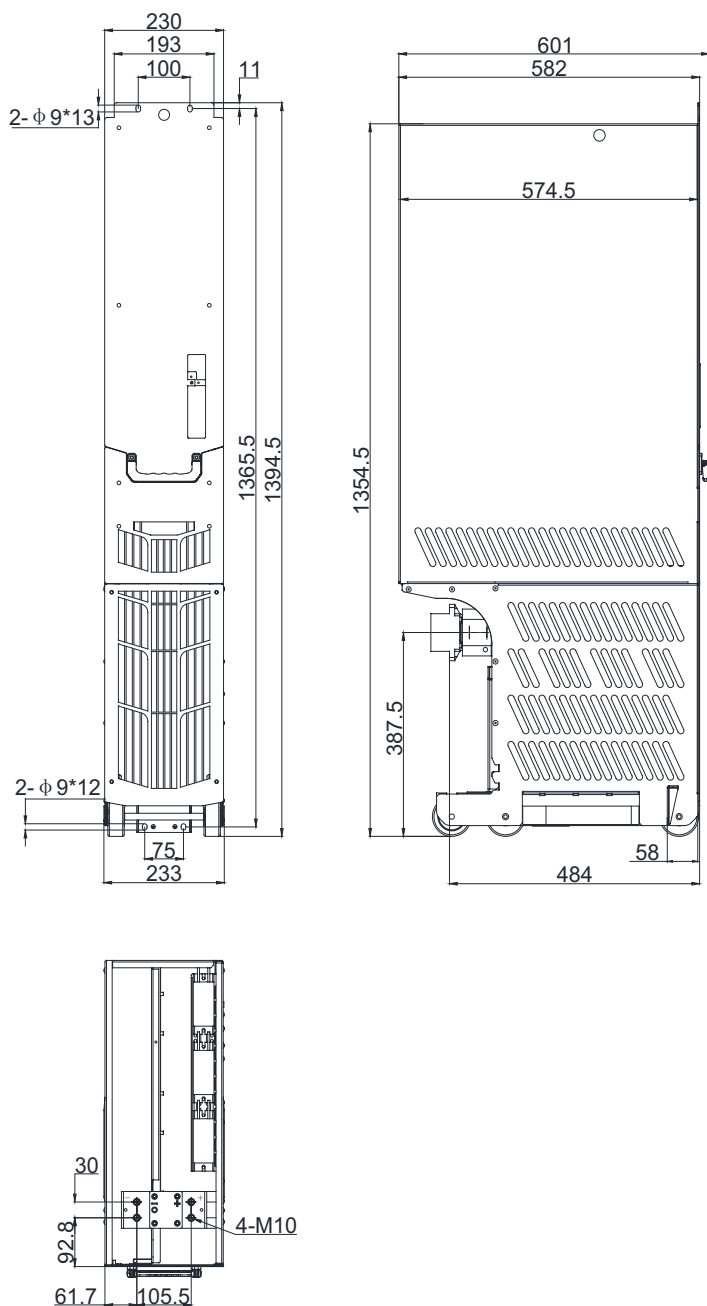
Рис. 2-22 Габариты инвертора Н8 (мм)
