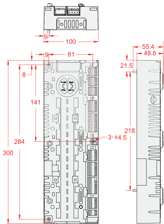
Рис. 5-2. Модуль HCU
