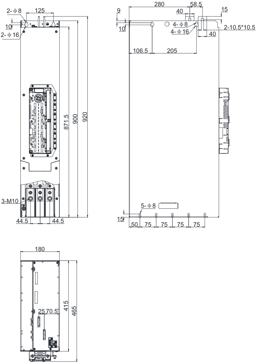
Рис. 2-21 Габариты инвертора Н7 (мм)
