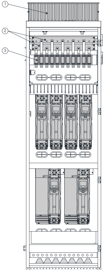
Рис. 3-8 Шкаф для Н1...Н4 – 600 мм
