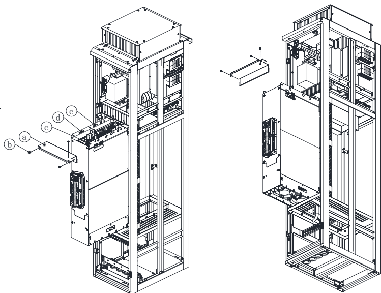
Рис. 7-6 Замена вентилятора инверторного блока типов размеров Н6...Н7
