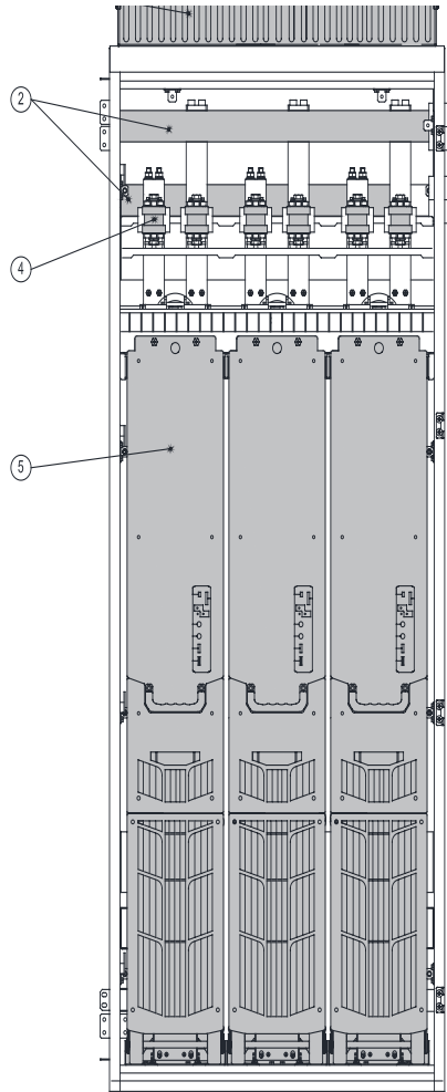
Рис. 3-19 Шкаф для Н8 – 800 мм
