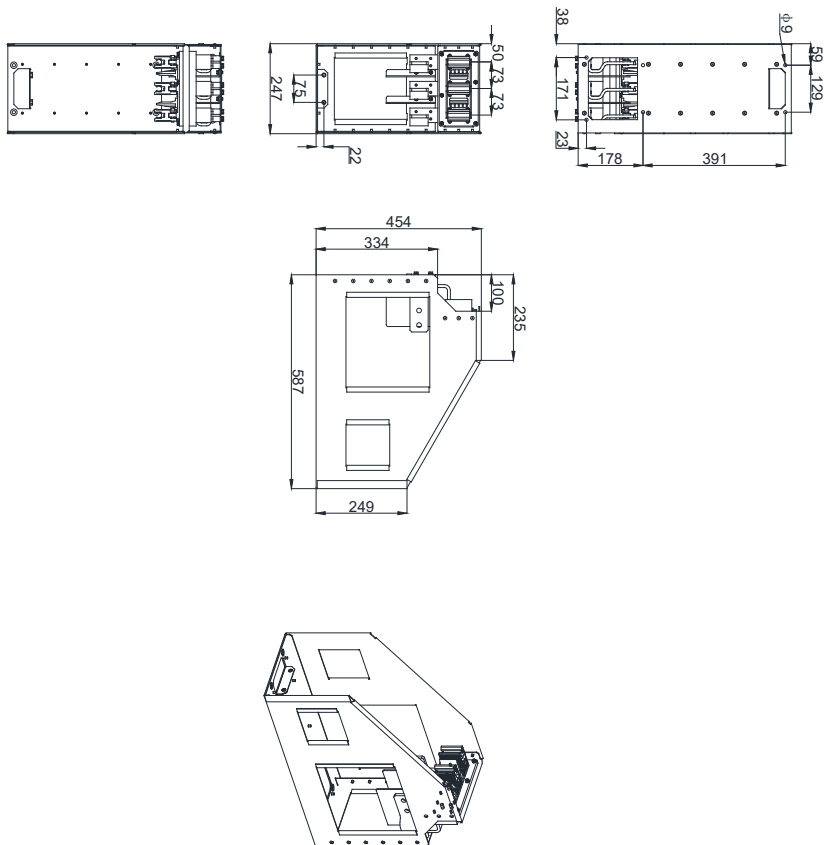
Рис. 8-10 Размеры комплекта для быстрой установки H8-quick-kit
