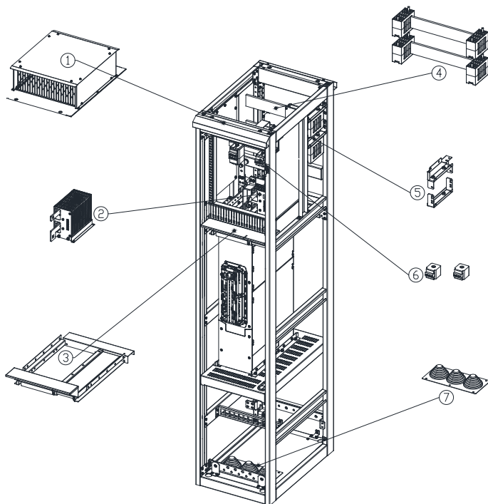
Рис. 3-12 Установка компонентов Н6...Н7 в шкаф 400 мм
