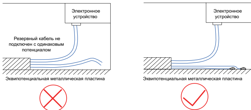
Рис. 4-5 Обращение с неиспользуемыми жилами многожильного кабеля
