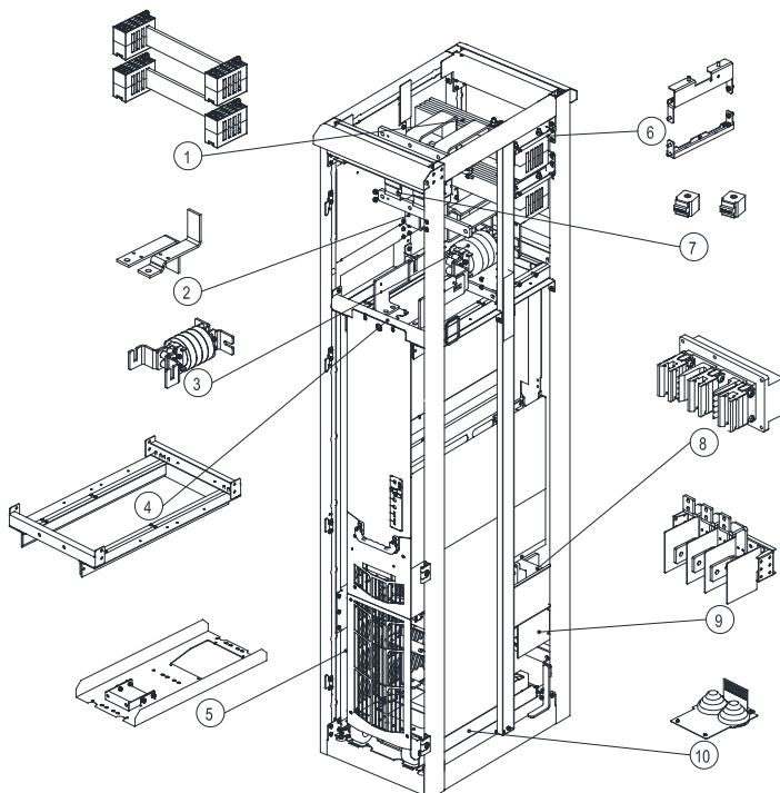
Рис. 3-15 Компоновка шкафа Н8 – 400 мм (только предохранитель)
