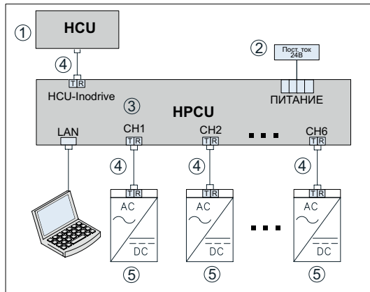
Рис. 5-8 Схема электрического подключения НРСУ
