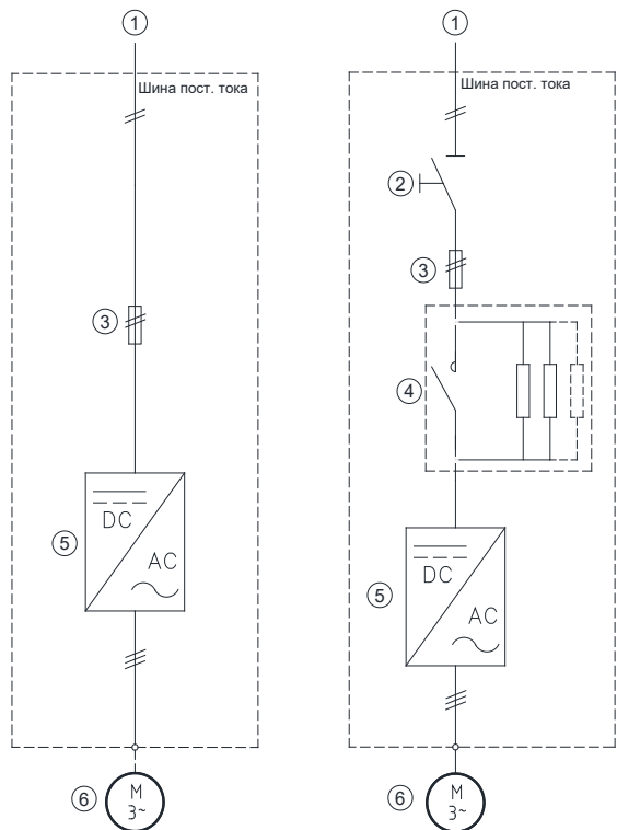
Рис. 2-13 Схема электрического подключения Н7
