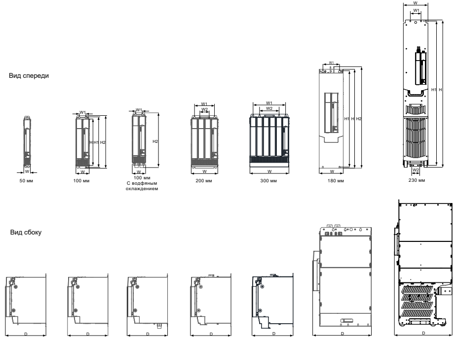
Рис. 1-3 Габаритные размеры привода (одноосевой)
