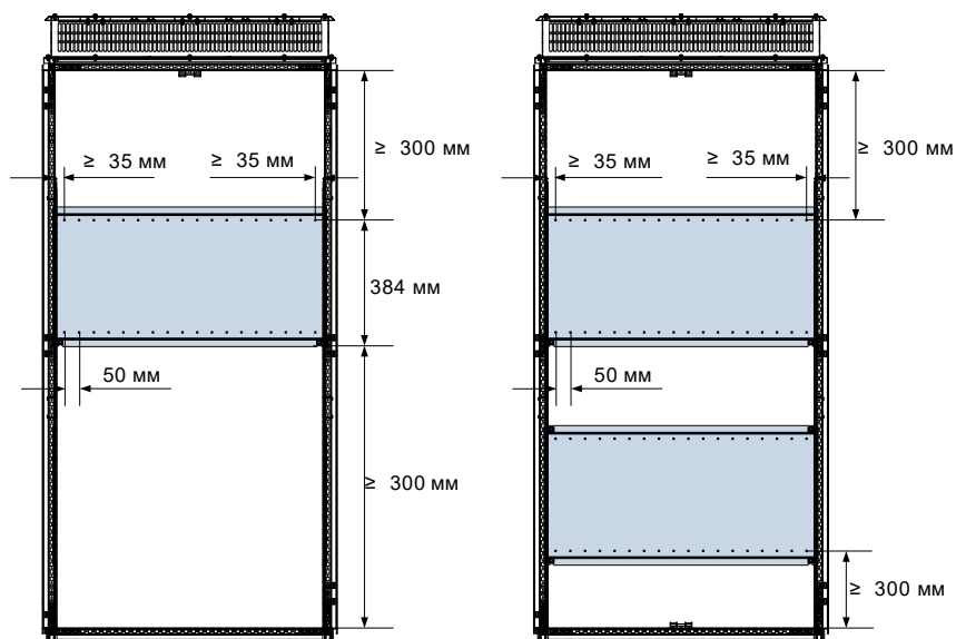
Монтаж в одиночной стойке
