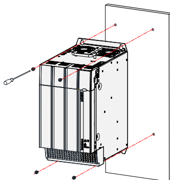
Рис. 2-3 Монтаж задней панели MD810-50M4T45G—MD810-50M4T75G
