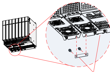
Алюминиевый стержень заземления ЭМС (поставляется вместе с оборудованием) для соединения всех блоков
