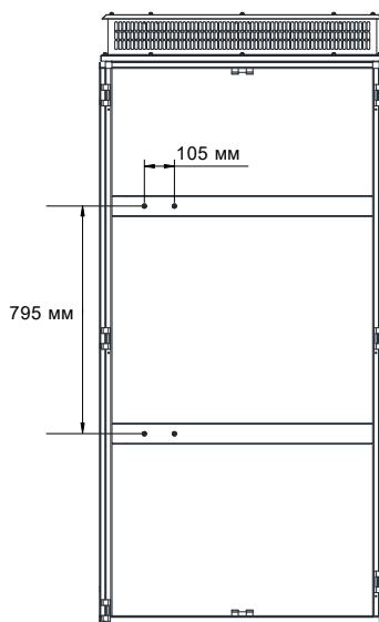
Монтаж на двух стойках
