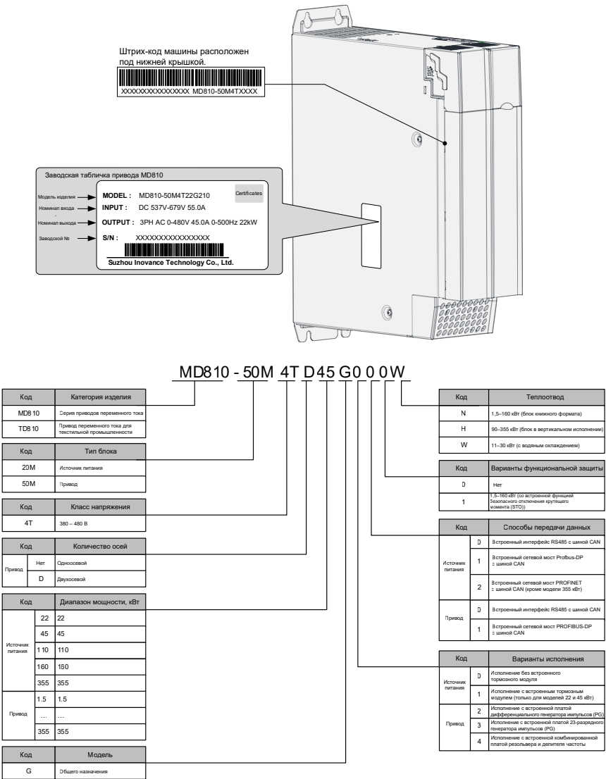
Рис. 1-1 Заводская табличка и код привода
