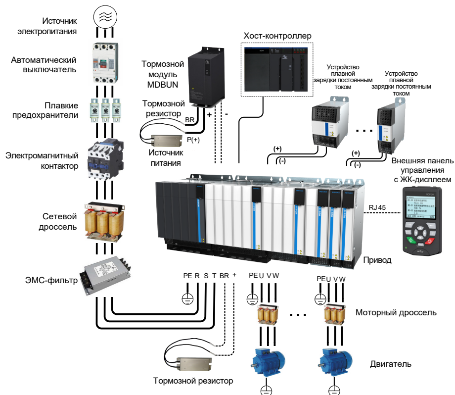
Рис. 1-5 Структура системы
