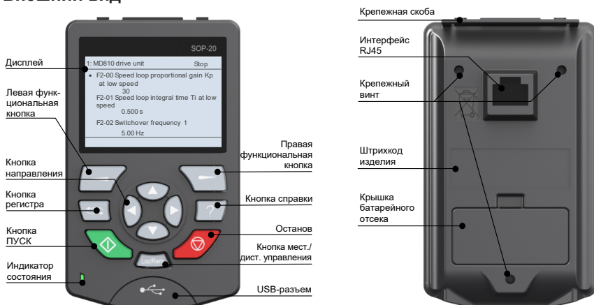
Рис. 4-3 Вид внешней панели управления с ЖК-дисплеем
