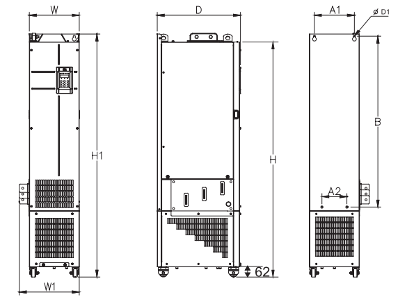
Габаритные и установочные размеры MD290 200G/220P-450G/500P (с дросселем)
