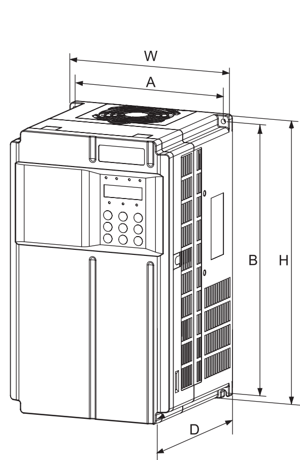
Габаритные и установочные размеры MD290 200G/220P-450G/500P (без дросселя)
