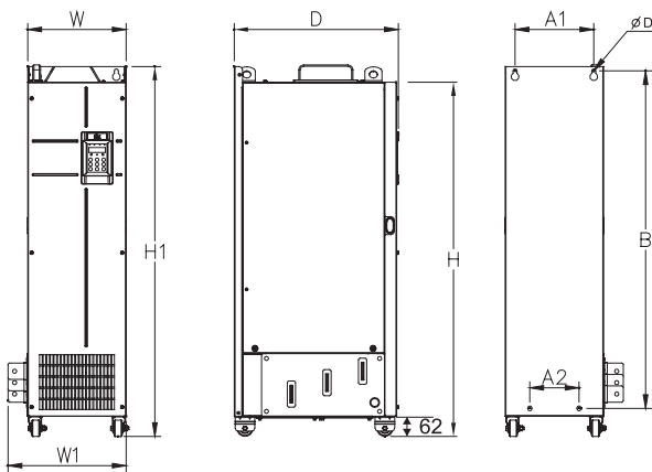
Габаритные и установочные размеры MD290 200G/220P-450G/500P (без дросселя)
